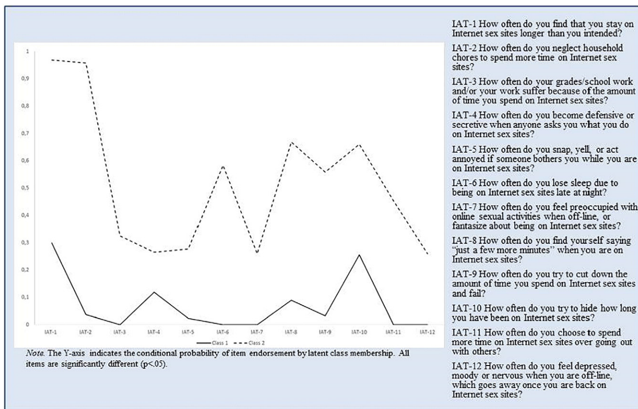
Fig. 1. Latent classes.
